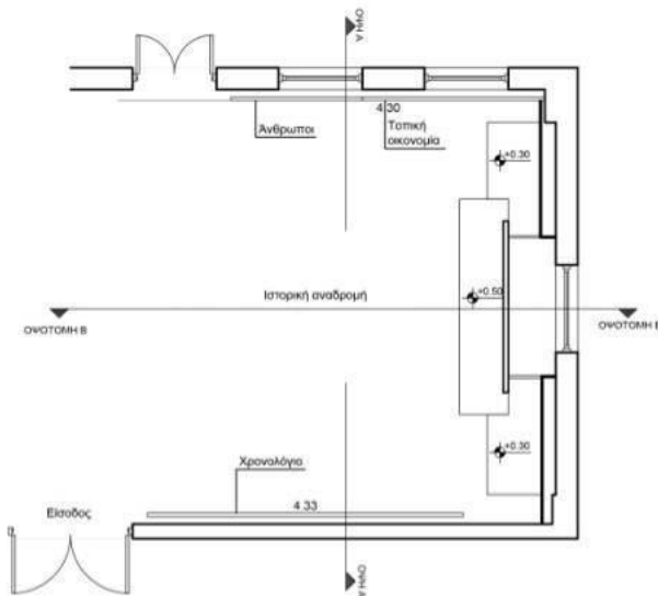
Γενική διάταξη - Κάτοψη τμήματος χώρου
